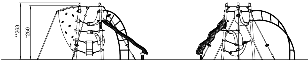
GXY802010 1:100
