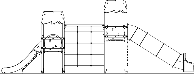
KPL4001-xx02 1:100
