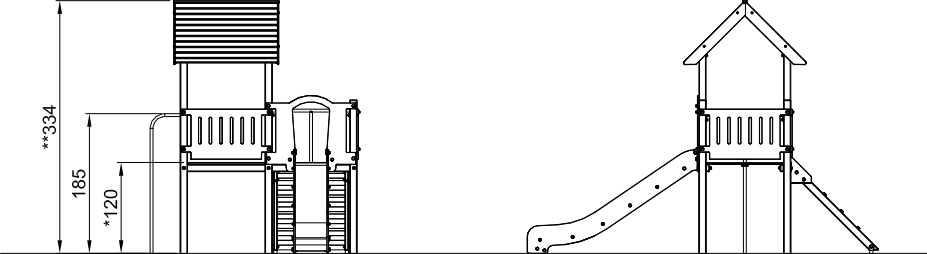
NAT1003 1:100
