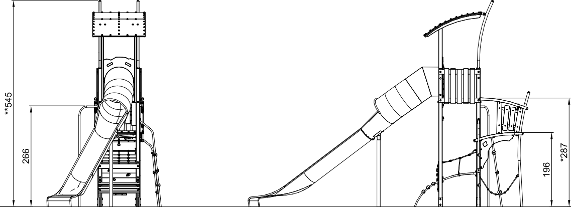
NAT520 1:100
